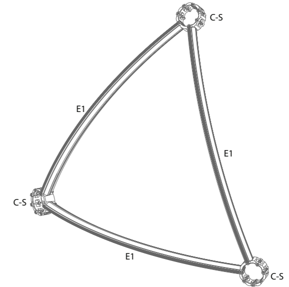
三角モジュール A180 M5 Triangular Module A180 M5
