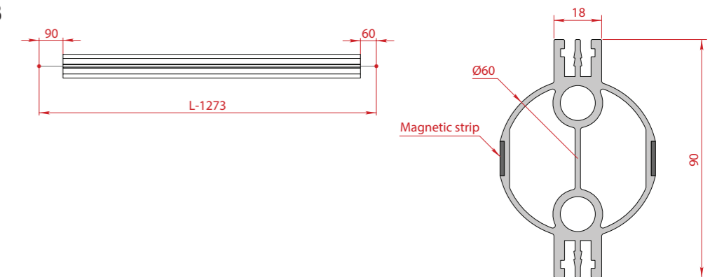
アルミ材 A180 E3 Aluminium Extrusion
