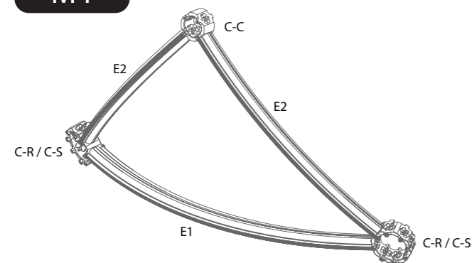
三角モジュール A180 M4 Triangular Module A180 M4
