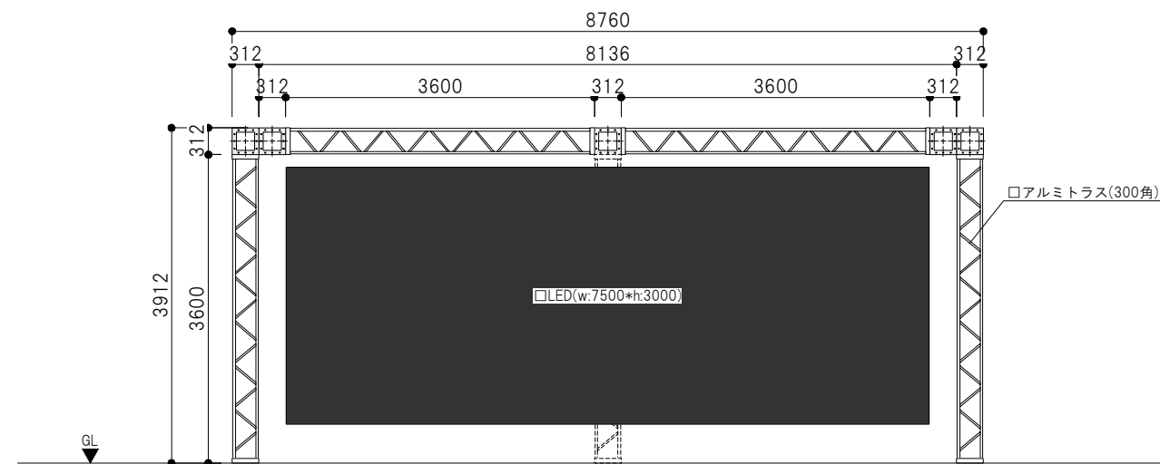
立面図A
