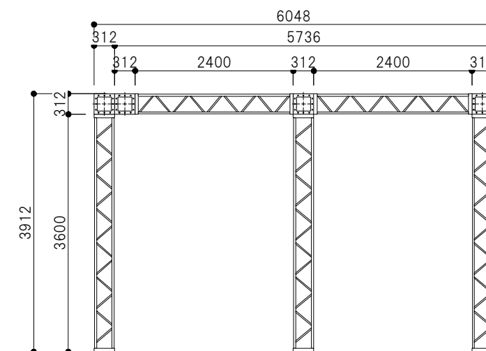
立面図D
