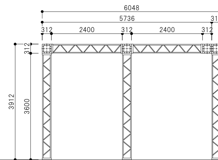
立面図B
