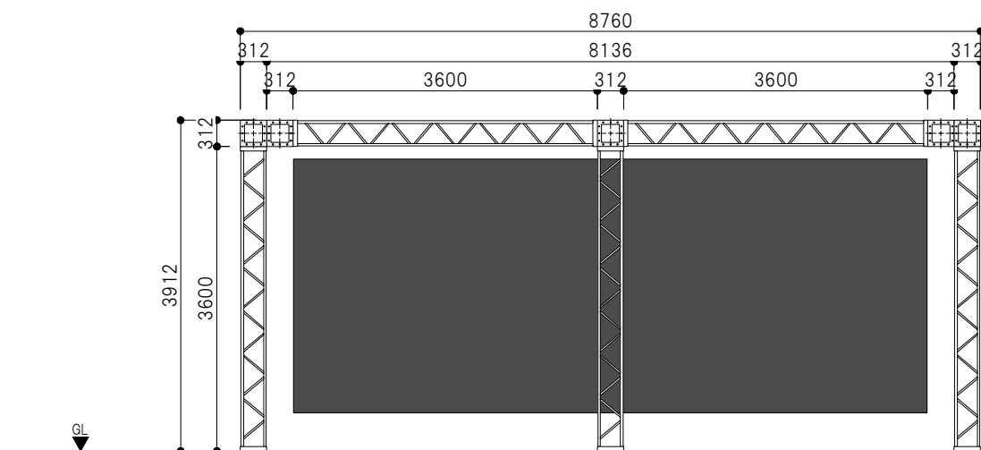
立面図C
