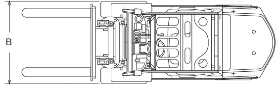
■主要寸法図
